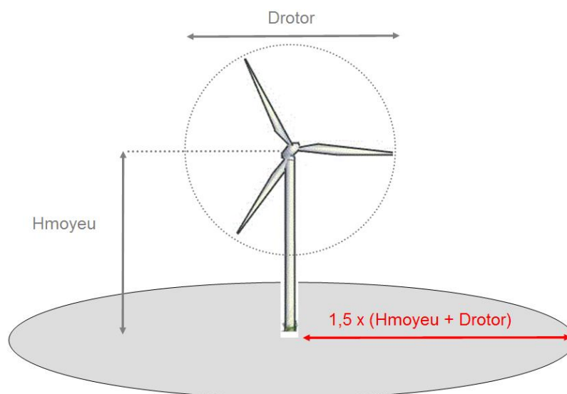
Figure 30 : Projection de glace — Schéma de principe de la distance d'effet
