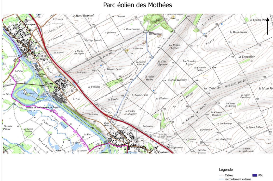
Figure 6 : Hypothèse de raccordement du projet au poste source de la Chaussée
