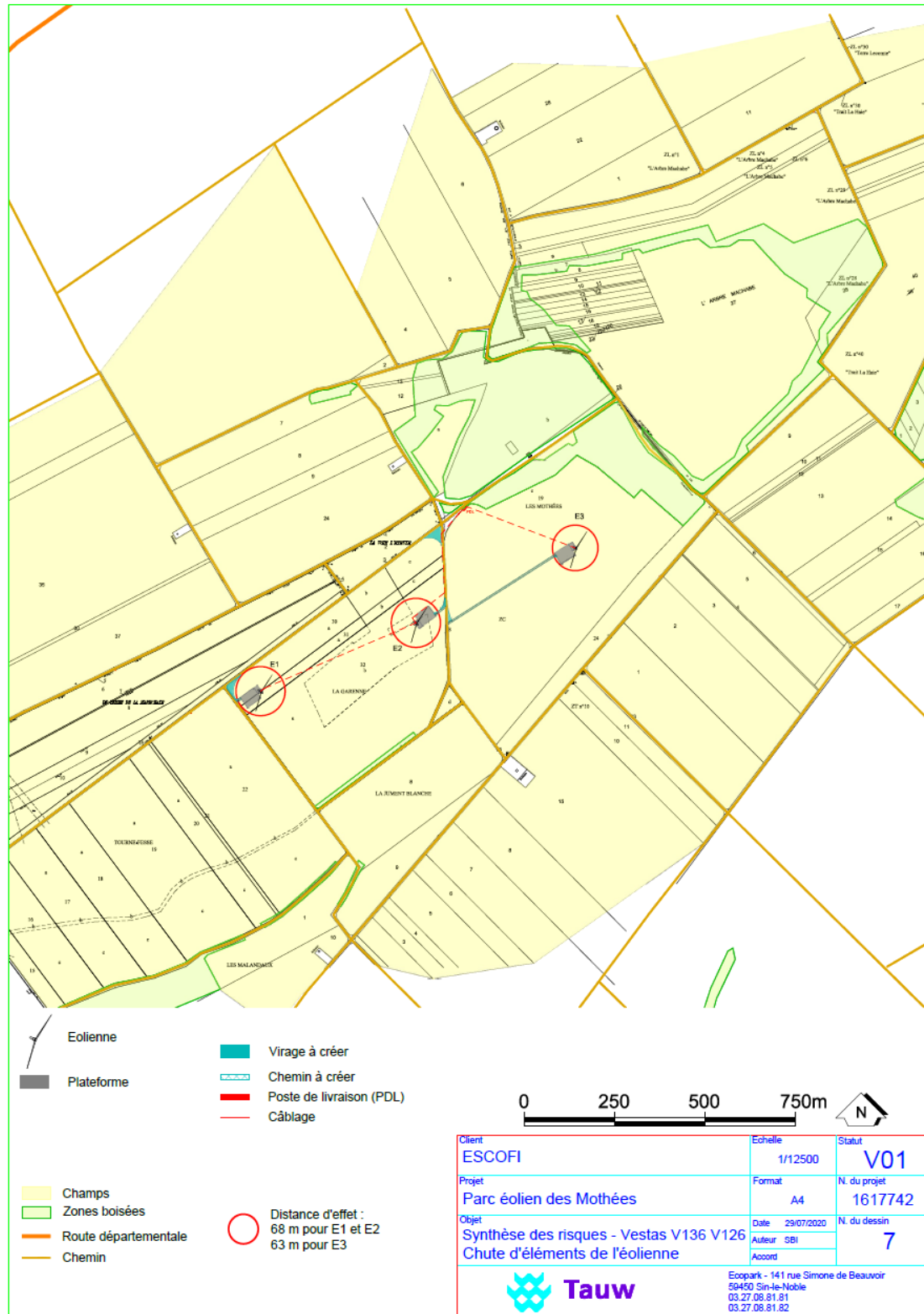
Figure 26 : Chute d'éléments de l'éolienne – carte des distances d'effet – scénario 2
