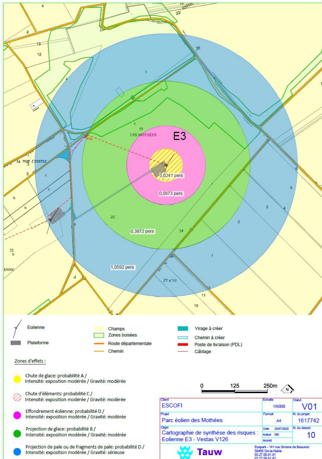
Figure 38 : Cartographie de synthèse des risques – E3 –scénario 2
