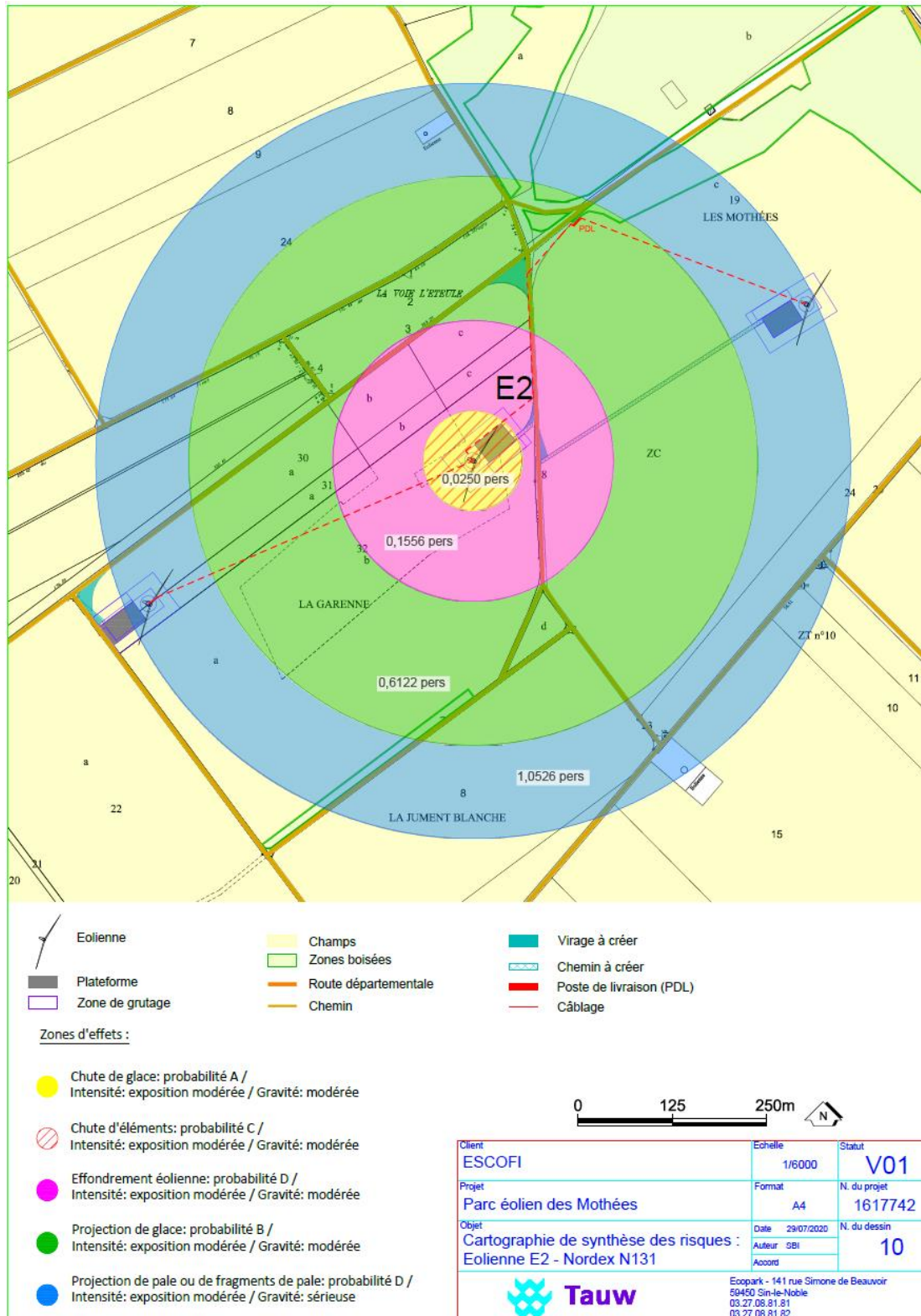
Figure 35 : Cartographie de synthèse des risques – E2 –scénario 1
