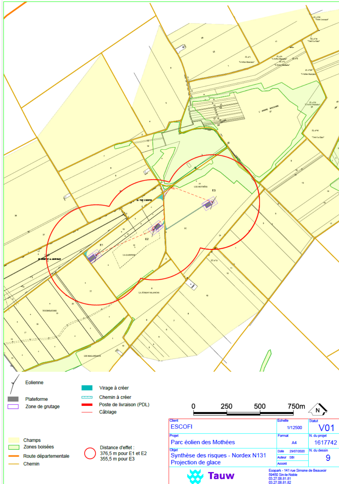
Figure 31 : Projection de morceaux de glace – carte des distances d'effets – scénario 1
