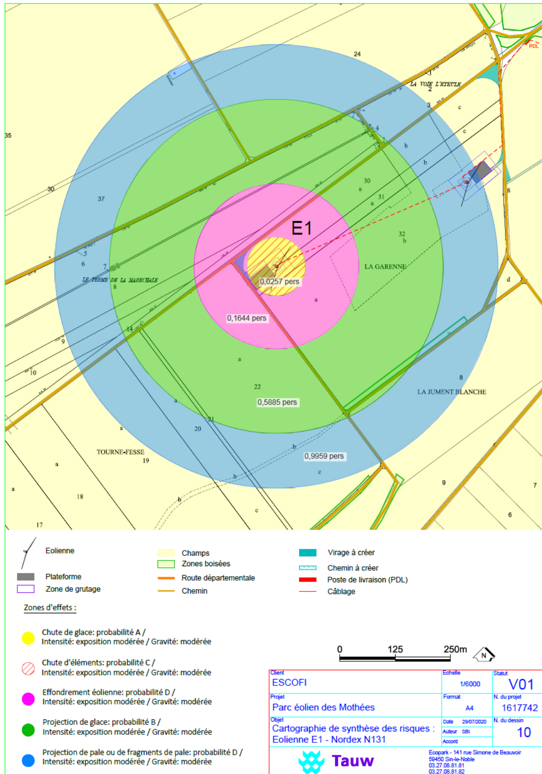
Figure 33 : Cartographie de synthèse des risques – E1 –scénario 1
