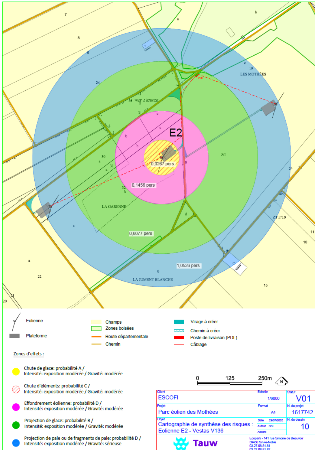
Figure 36 : Cartographie de synthèse des risques – E2 – scénario 2
