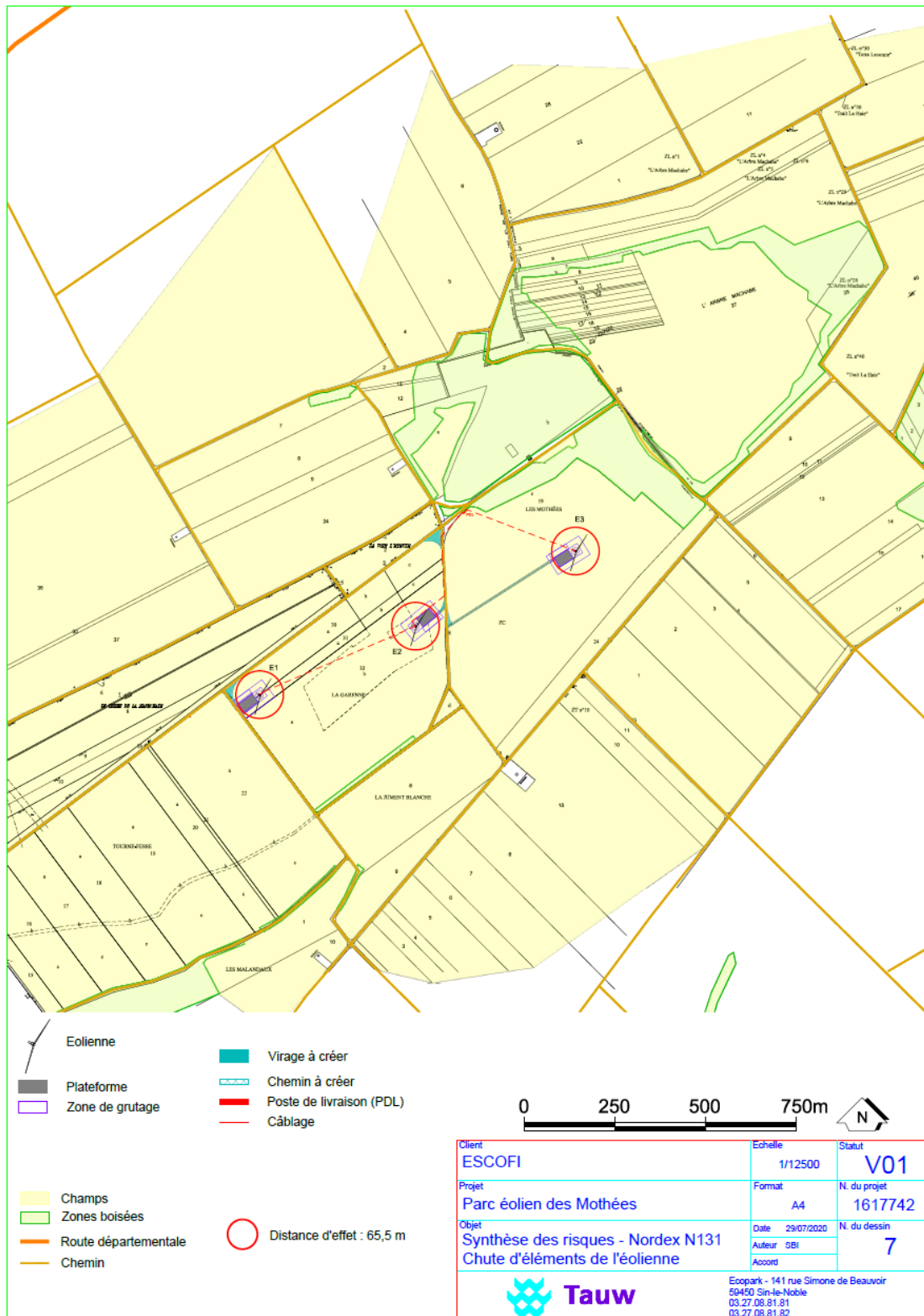
Figure 25 : Chute d'éléments de l'éolienne – carte des distances d'effet – scénario 1
