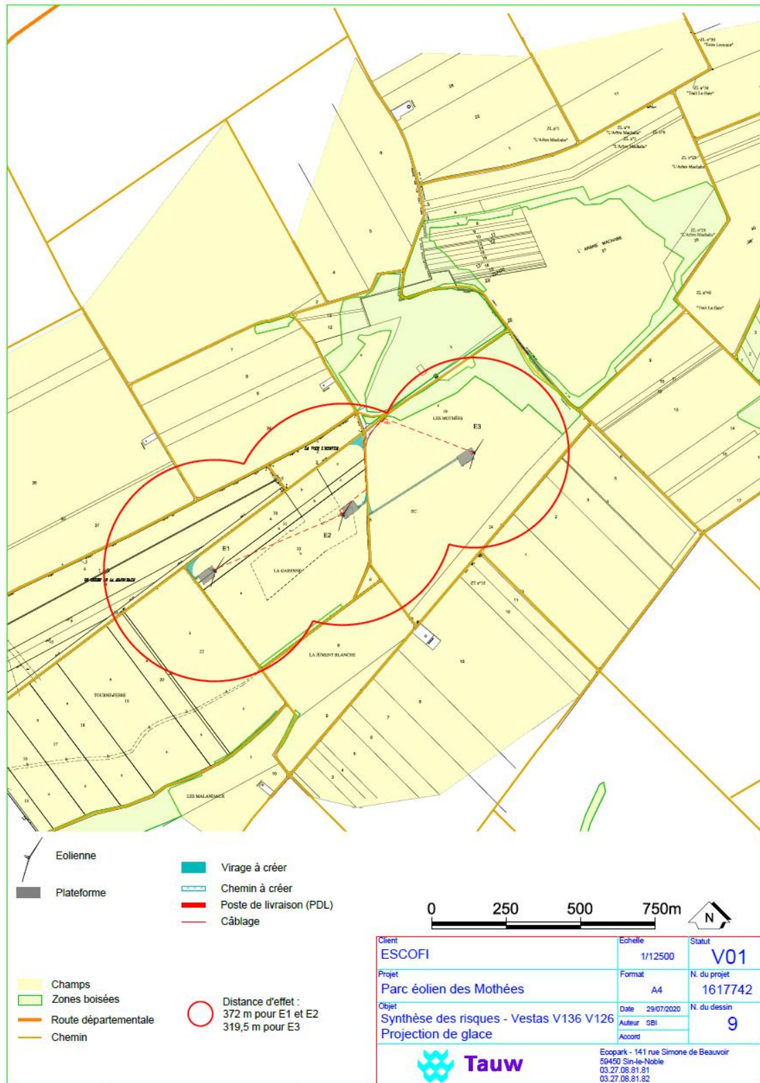
Figure 32 : Projection de morceaux de glace – carte des distances d'effets – scénario 2
