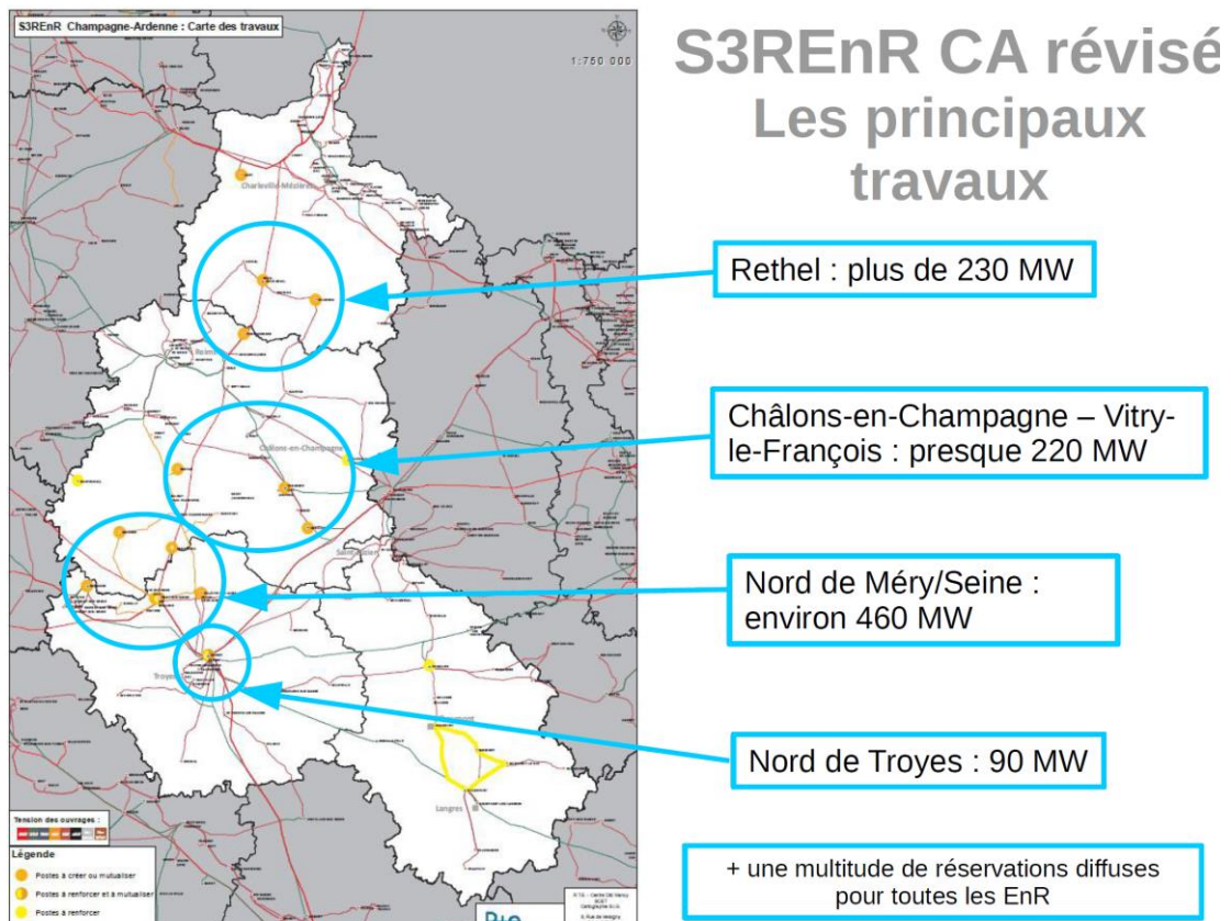
Figure 7 : Travaux retenus du S3REnR – Source : DREAL Grand-Est
