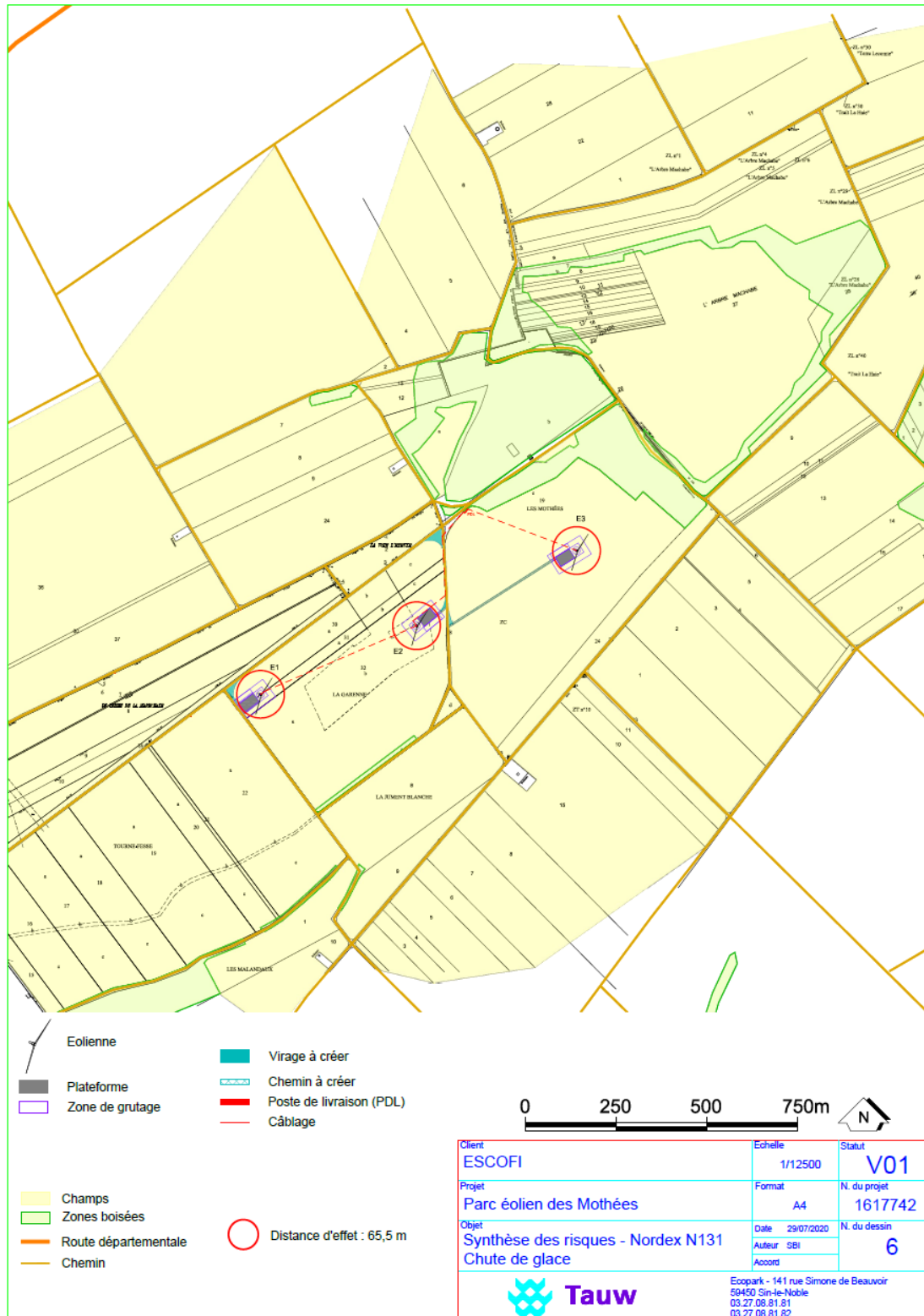
Figure 21 : Chute de glace – carte des distances d'effets – scénario 1
