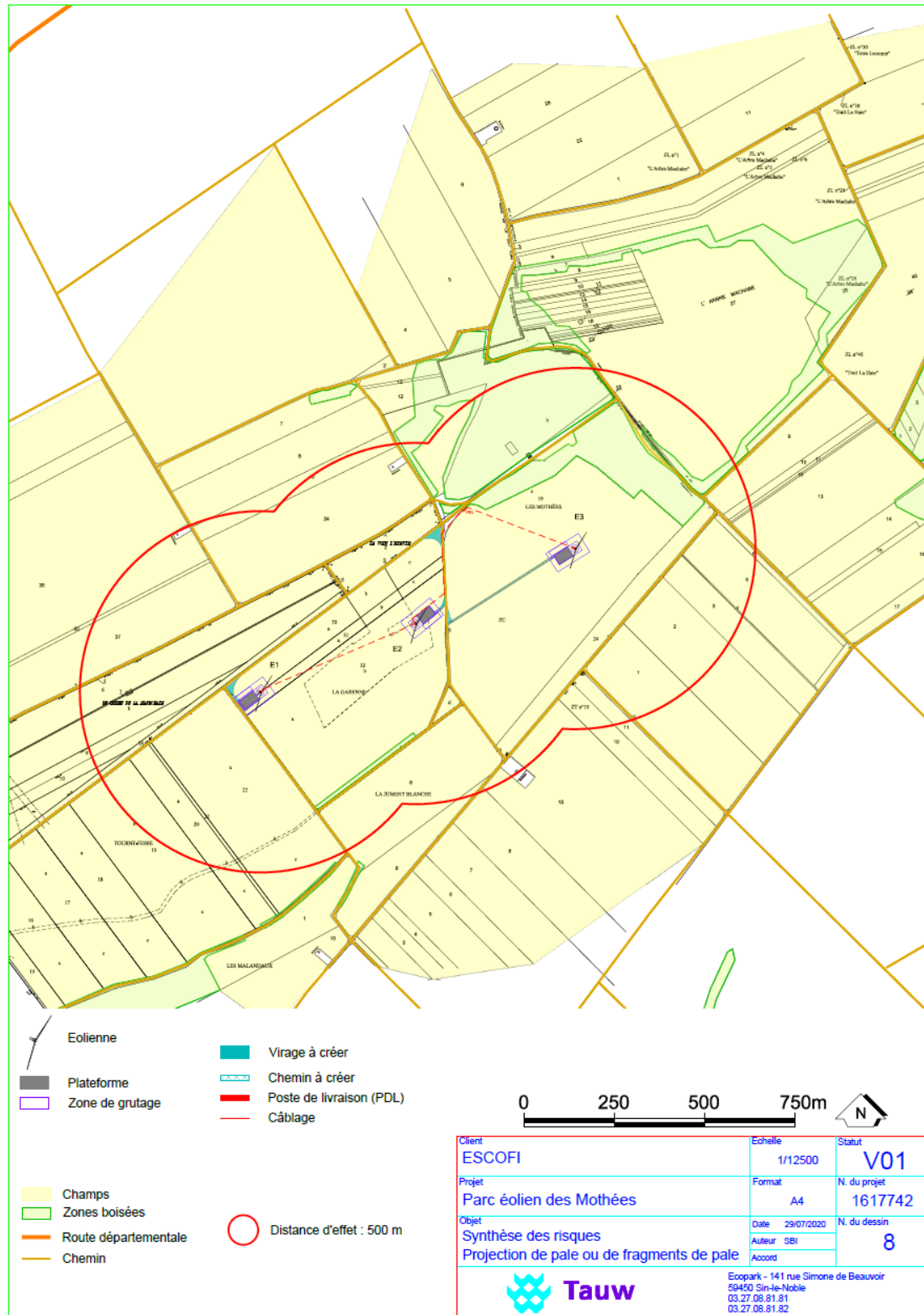
Figure 29 : Projection de pales ou de fragments de pale – carte des distances d'effets – scénario 1 et scénario 2
