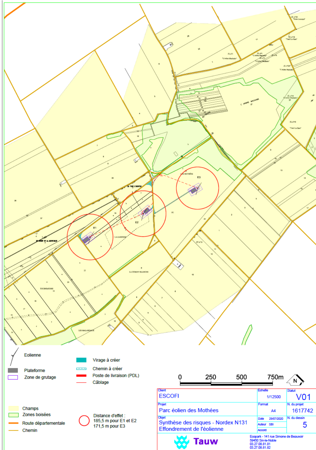
Figure 18 : Effondrement de l'éolienne – carte des distances d'effets – scénario 1
