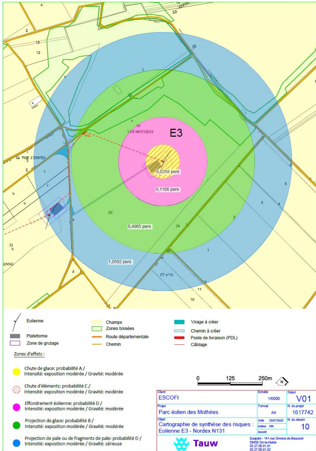
Figure 37 : Cartographie de synthèse des risques – E3 –scénario 1
