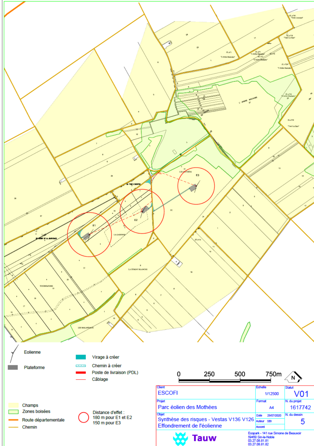
Figure 19 : Effondrement de l'éolienne – carte des distances d'effets – scénario 2
